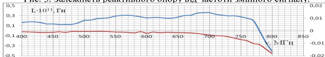
Рис. 4. Залежність еквівалентної індуктивності тиристора від частоти змінного сигналу (1- без зміщення; 2- U_{зм} = 0,5В ).
