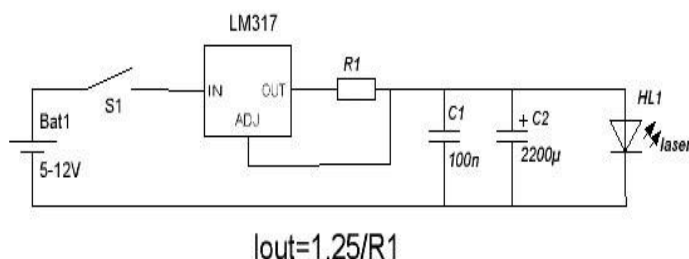
Рис. 1 Стабілізатор струму для лазерного діода.
