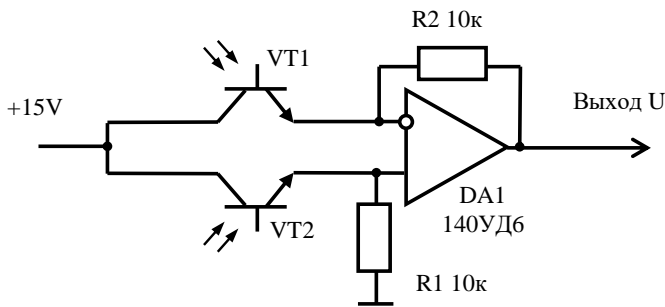
Рис.2. Схема дифференциального усилителя фототоков
