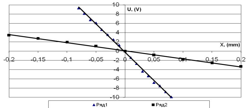
Рис.3. Зависимость выходного напряжения фотодатчиков от координаты падающего луча. Ряд 1 – два отдельных фототранзистора, освещаемых лазером. Ряд 2 – спаренный фототранзистор, освещаемый лампой накаливания микроскопа.
