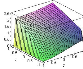
Рис.6 График функции \Lambda(x, y)
