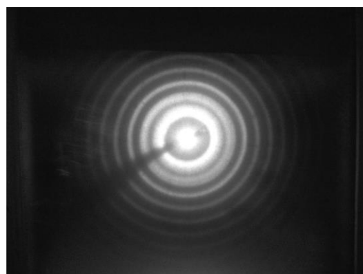
Рис.4. Хвилі від точкового джерела з частотою коливань 80 \text{ Гц}
