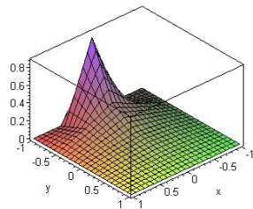
Рис.5 График функции N_3(x, y)
