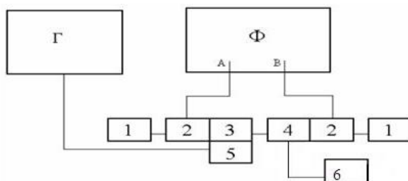
Рис. 1. Структурна схема експериментальної установки на базі фазометра ФК2-12. (Ф – вимірювач різниці фаз ФК2-12; Г – генератор; 1 – коаксіальне навантаження; 2 – трійник ТП-1; 3 – трійник ТН, 4 – досліджуваний чотириполюсник; 5 – трійник ТС; 6 – стабілізоване джерело живлення, Б5-50;).
